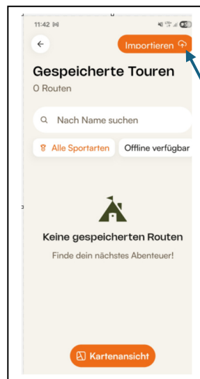
Fig. 3.1: 4. GPS data
